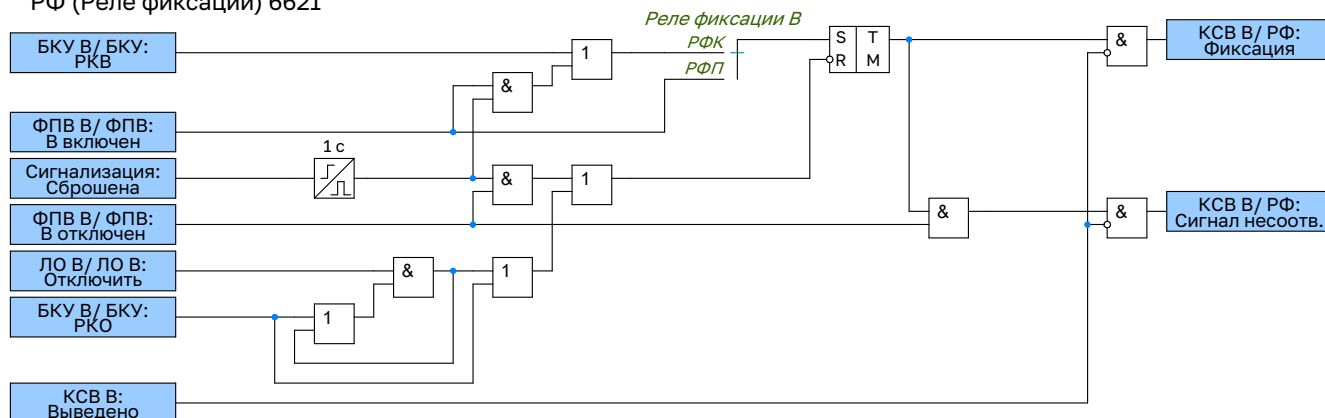
Рисунок 2.34 – Функциональная схема логики реле фиксации выключателя
