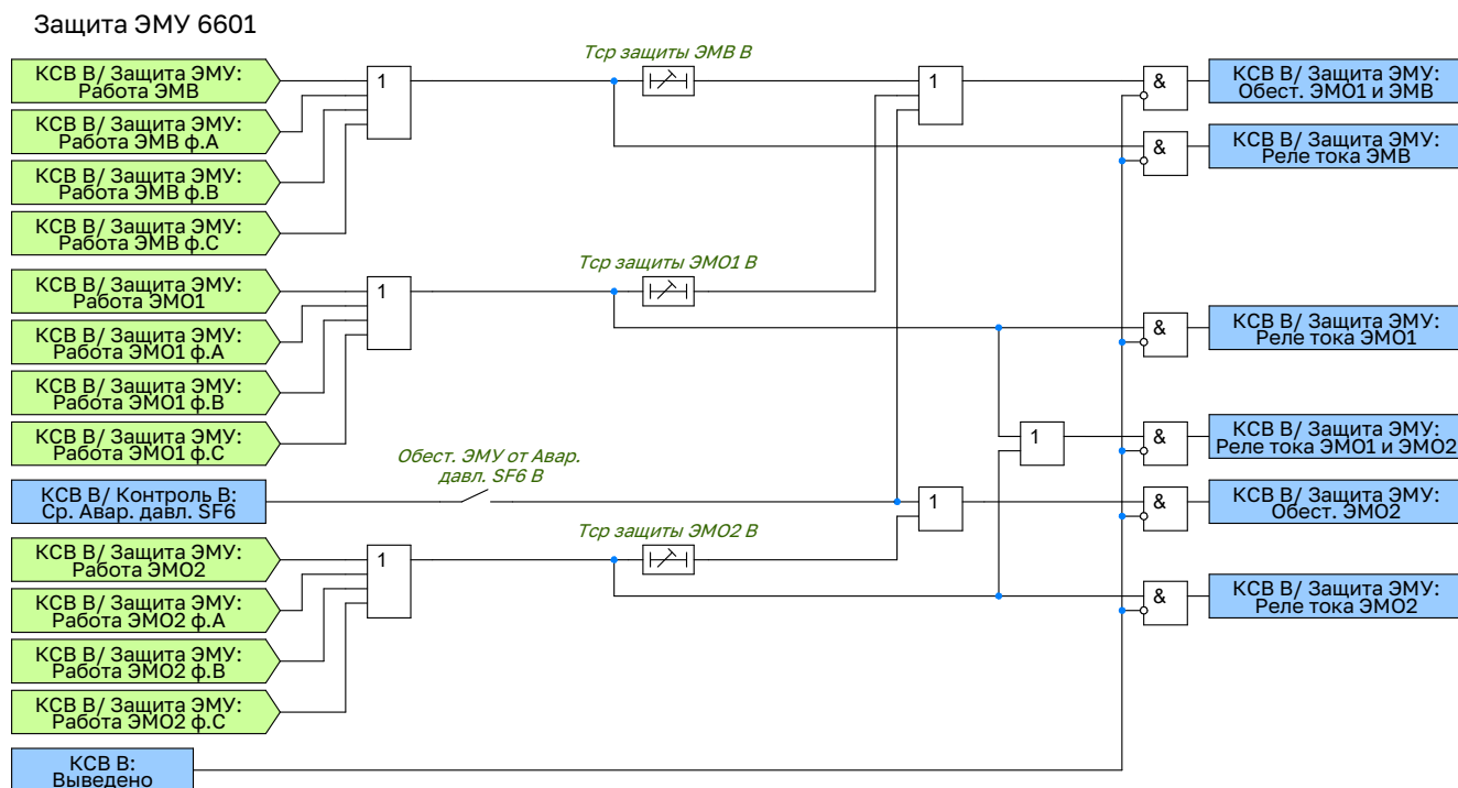
Рисунок 2.32 – Функциональная схема логики защиты ЭМУ выключателя
