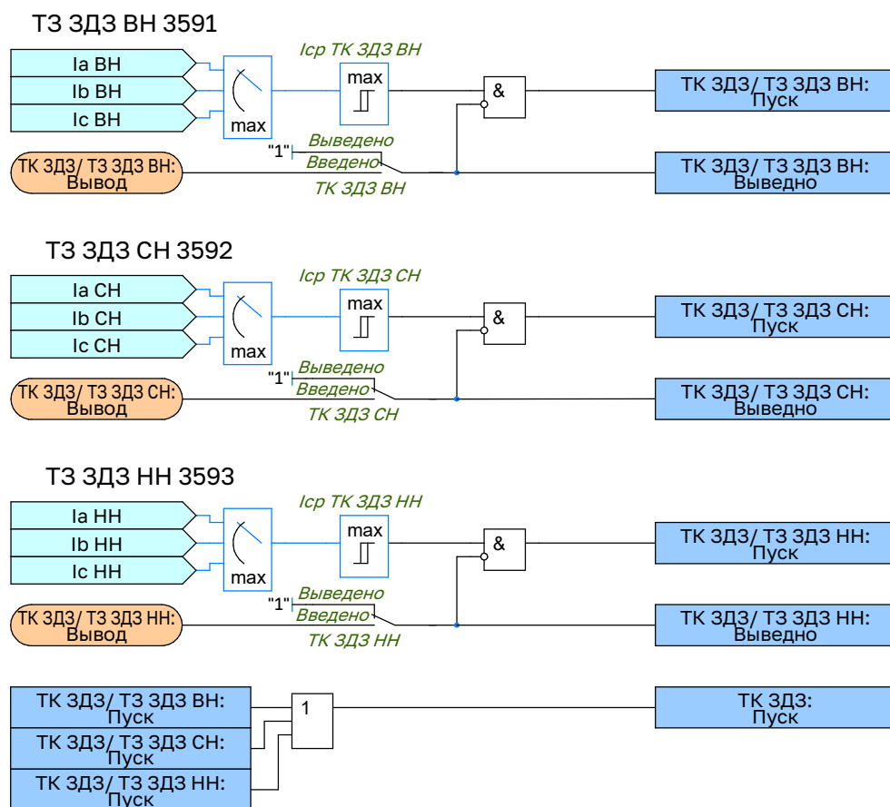
Рисунок 2.15 – Функциональная схема логики ТК ЗДЗ
