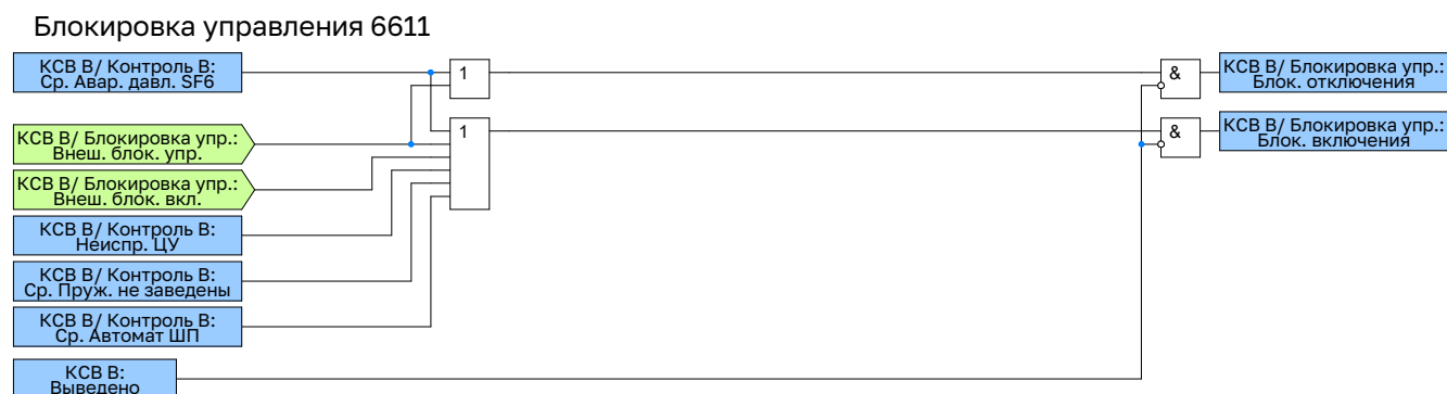
Рисунок 2.33 – Функциональная схема логики блокировки управления выключателя
