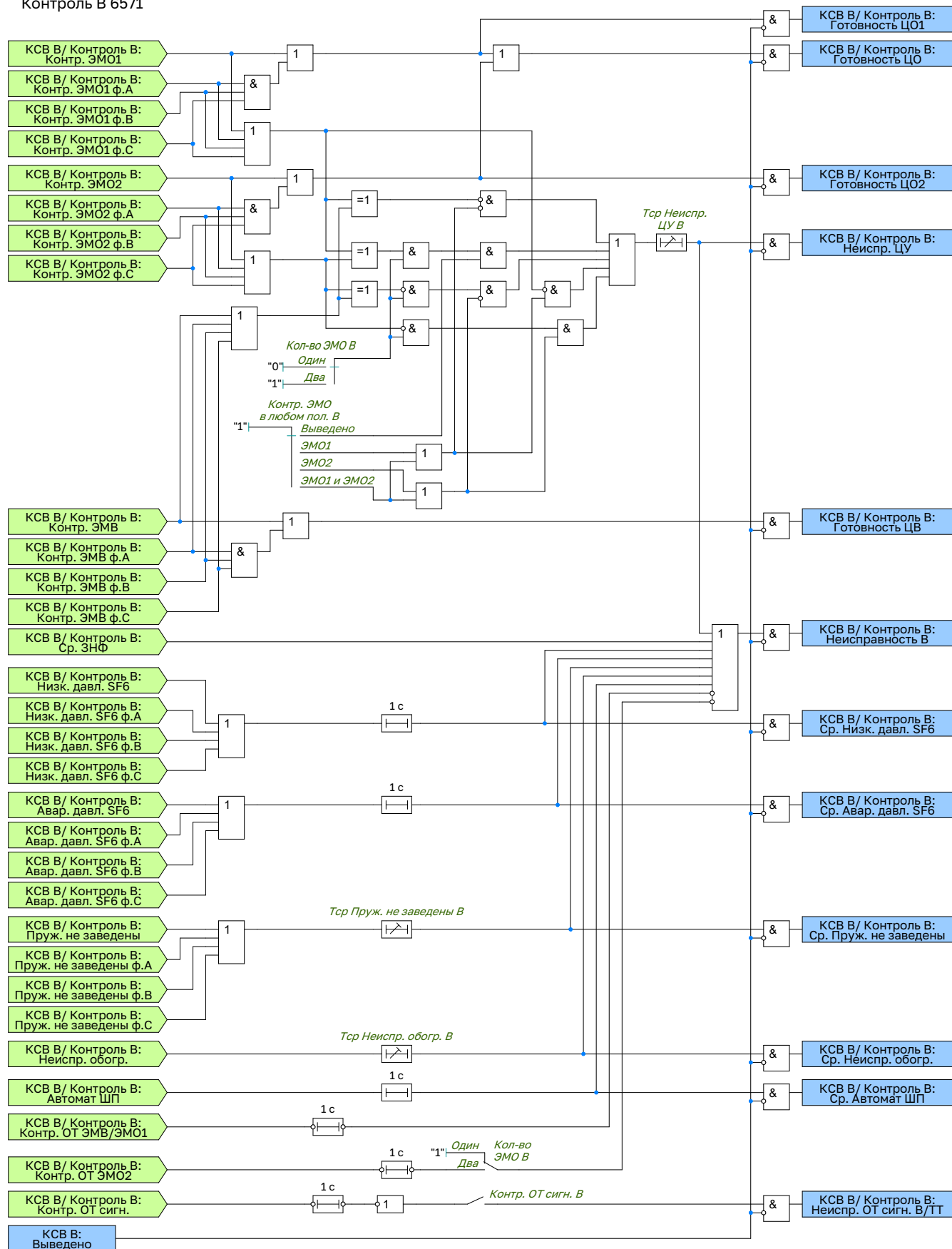
Рисунок 2.30 – Функциональная схема логики контроля выключателя
