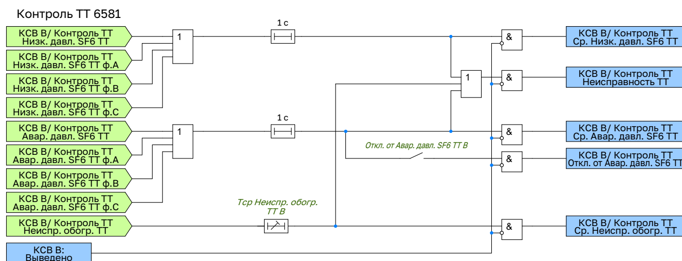
Рисунок 2.31 – Функциональная схема логики контроля ТТ выключателя
